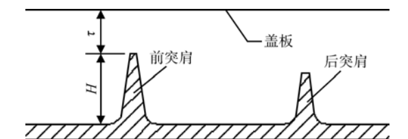
图 7 叶尖间隙示意图
