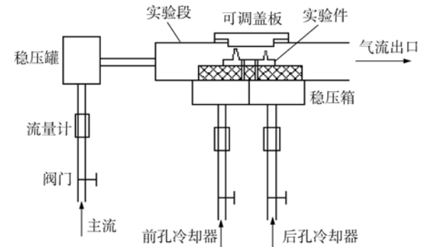
图 6 实验系统图
