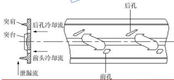
图 5 模型平面图
