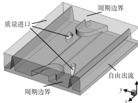
图 2 计算域及边界条件
