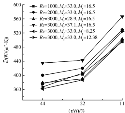
图16 平均表面传热系数随叶尖间隙变化曲线
