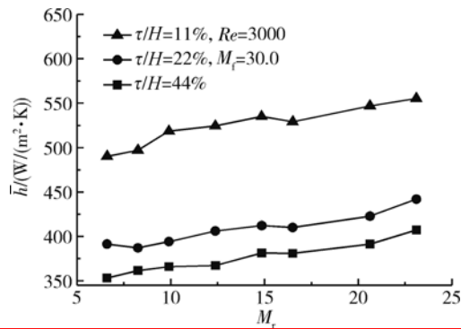
图13 平均表面传热系数随后孔出流比变化曲线
