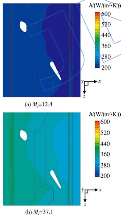
图14 不同前孔出流比下叶冠的表面传热系数云图
