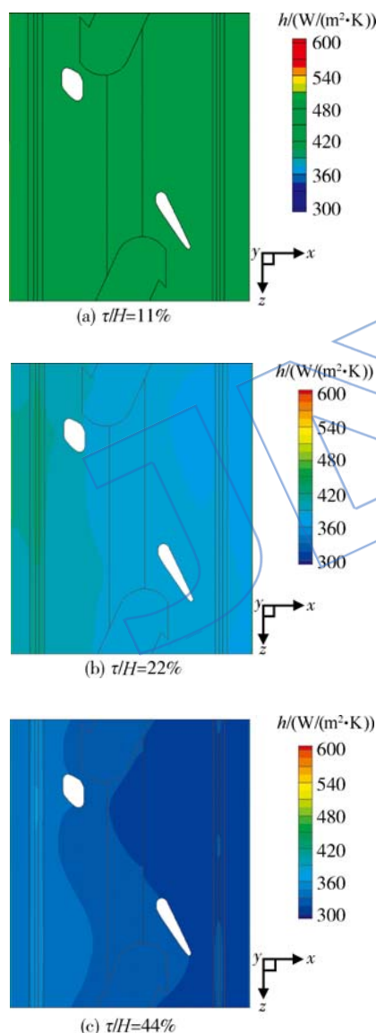
图 17 不同叶尖间隙下叶冠的表面传热系数云图
